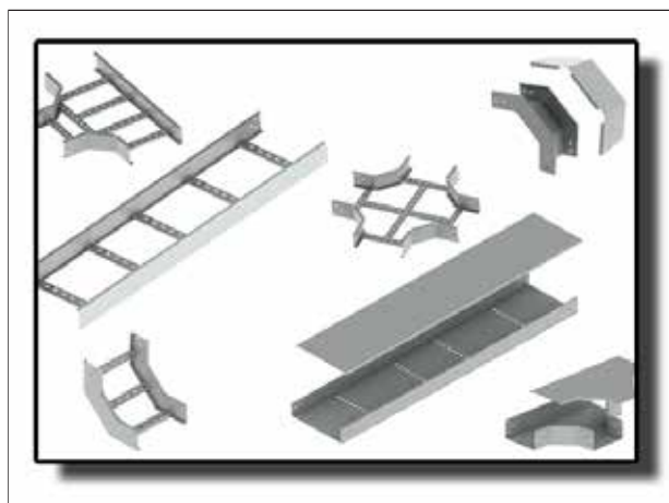
Thang & máng cáp Cable ladder & cable trays
