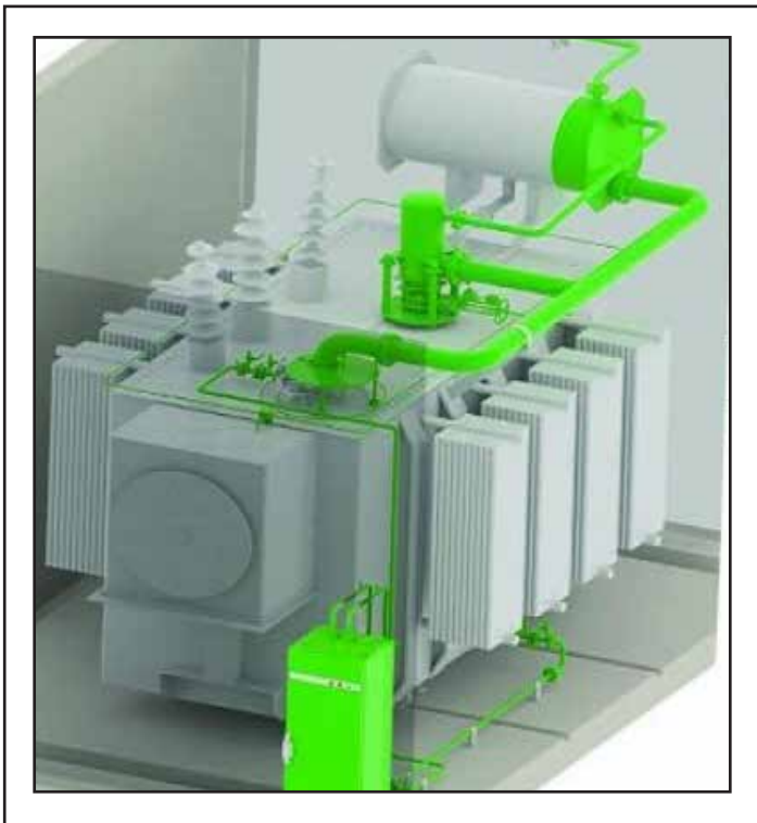
Thiết bị bảo vệ chống cháy nổ cho máy biến điện áp Transformer protector
